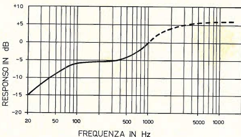
Fig. 1 - Grafico illustrante la curva di responso che è necessario conferire ad una testina ceramica, applicando un carico adatto ed una equalizzazione appropriata, affinché essa si presti alla riproduzione di dischi registrati in conformità alla curva RIAA.
