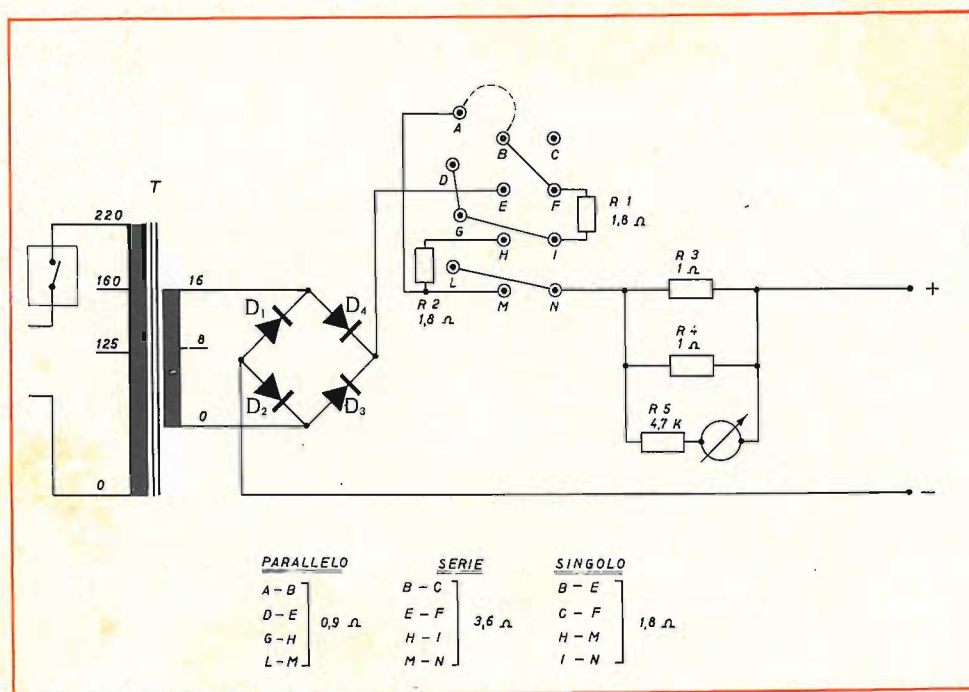
Fig. 1 - Schema elettrico del carica batterie
