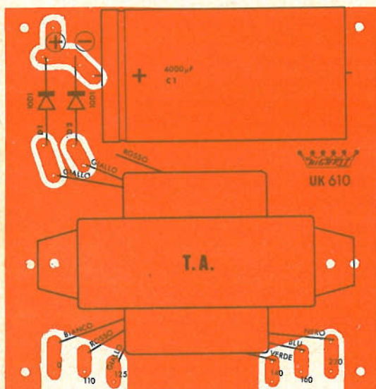
Fig. 2 - Serigrafia del circuito stampato UK 610.
