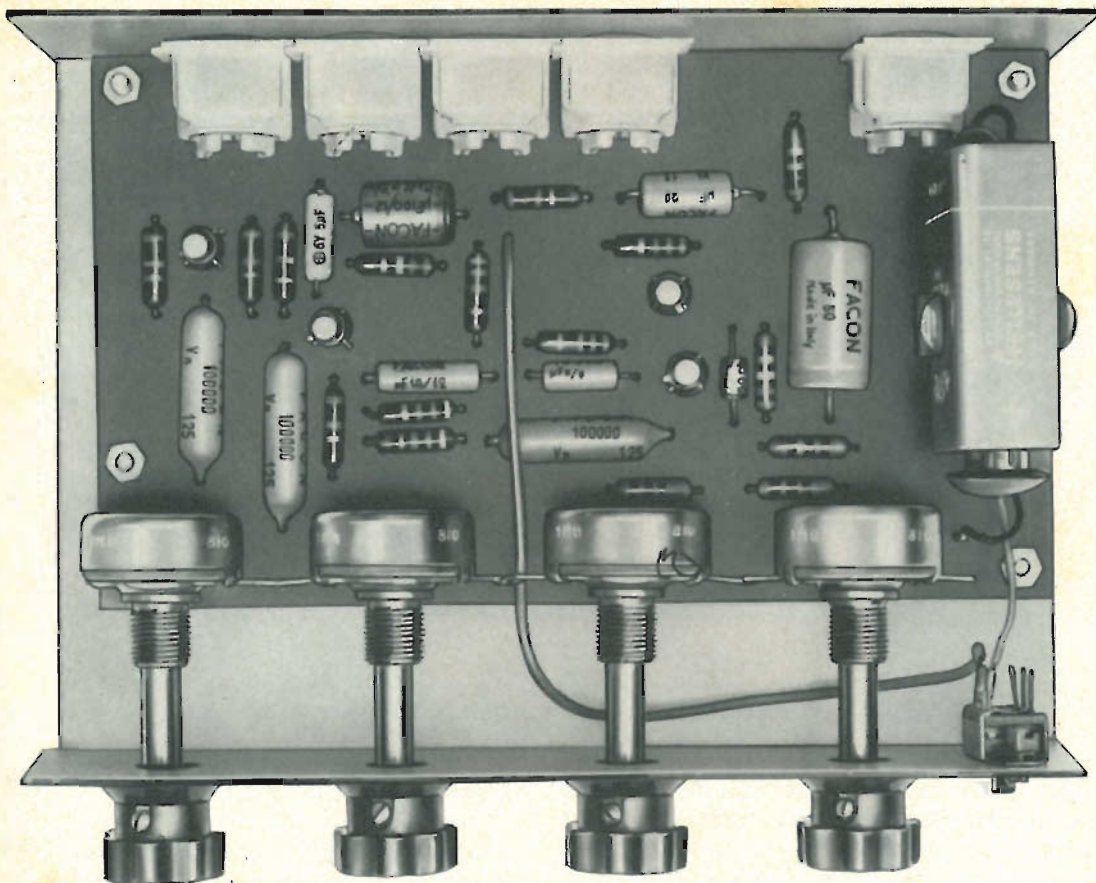
Fig. 4 - Aspetto dell'UK 710 a montaggio dei componenti ultimato.
