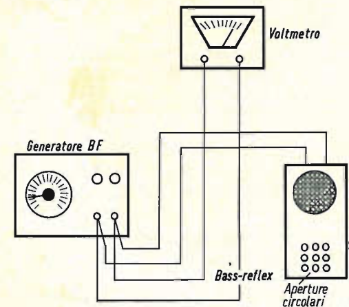
Fig. 1 - Circuito di principio per la determinazione dell'impedenza del sistema di altoparlanti. L'altoparlante è azionato direttamente dal generatore di bassa frequenza.
