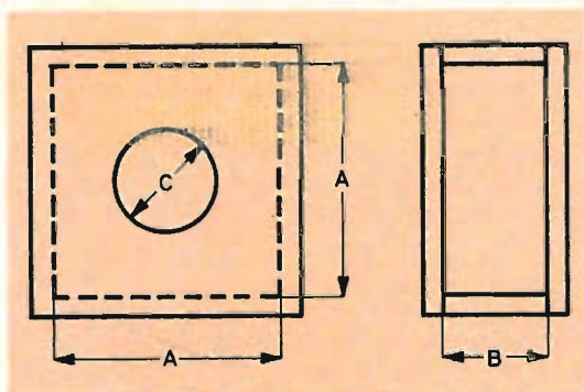
Disegno schematico quotato di una cassa acustica.
