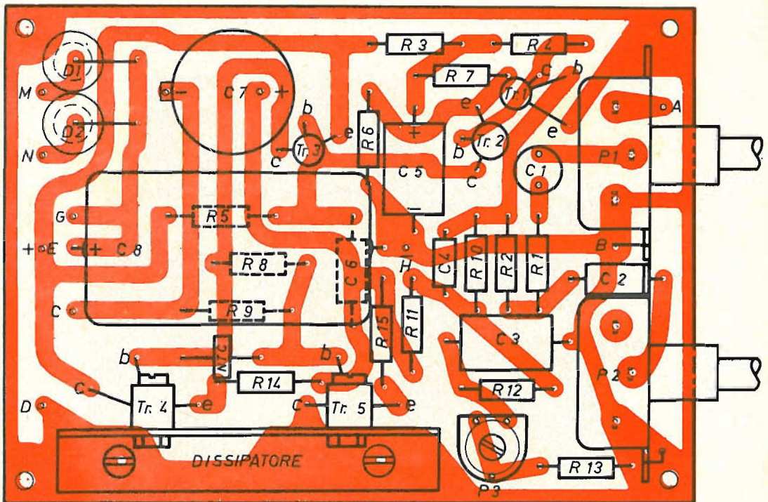
Fig. 2 - Disposizione dei componenti sulla faccia isolata del circuito stampato
