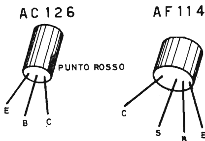
Fig. 3 - Come riconoscere i terminali dei due transistor impiegati.
