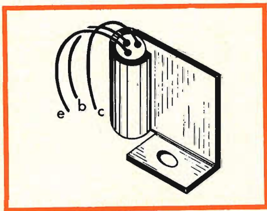
Fig. 3 - Disposizione del transistor TR 3 nel dissipatore.
