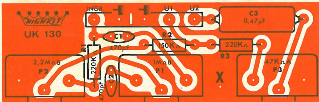
Fig. 2. - Serigrafia del circuito stampato
