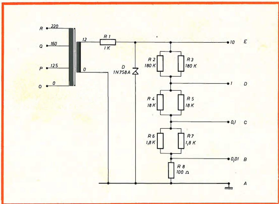
Fig. 1 - Schema elettrico.
