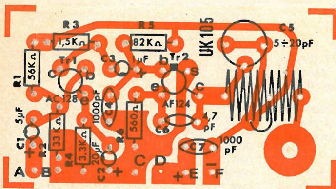
Fig. 2 - Disposizione dei componenti sulla piastra a circuito stampato.
