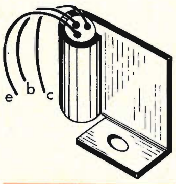
Fig. 5 - Come si devono piegare i terminali del transistor TR3 per il fissaggio sul dissipatore.
