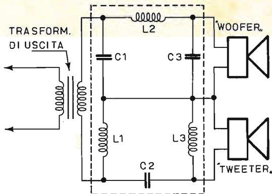
Fig. 2 - Il filtro « crossover » più semplice consiste soltanto nel collegare una capacità di valore adeguato in parallelo al « woofer », onde attenuare i segnali a frequenza acuta ai capi della sua bobina mobile, e diminuire la reattanza dell'intero circuito in serie rispetto al « tweeter ». Questo metodo — però — non consente di eliminare la dissipazione da parte del « tweeter » di una parte dell'energia dei segnali a frequenza bassa.
