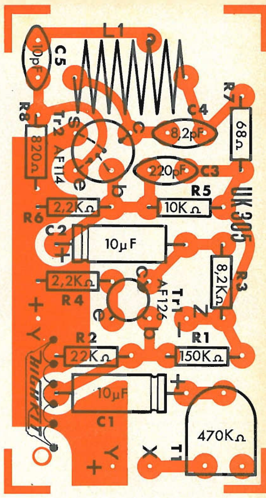
Fig. 2 - Disposizione dei componenti sulla piastra a circuito stampato.
