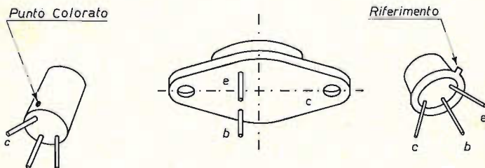
Fig. 1 - Disposizione dei terminali dei transistor.
