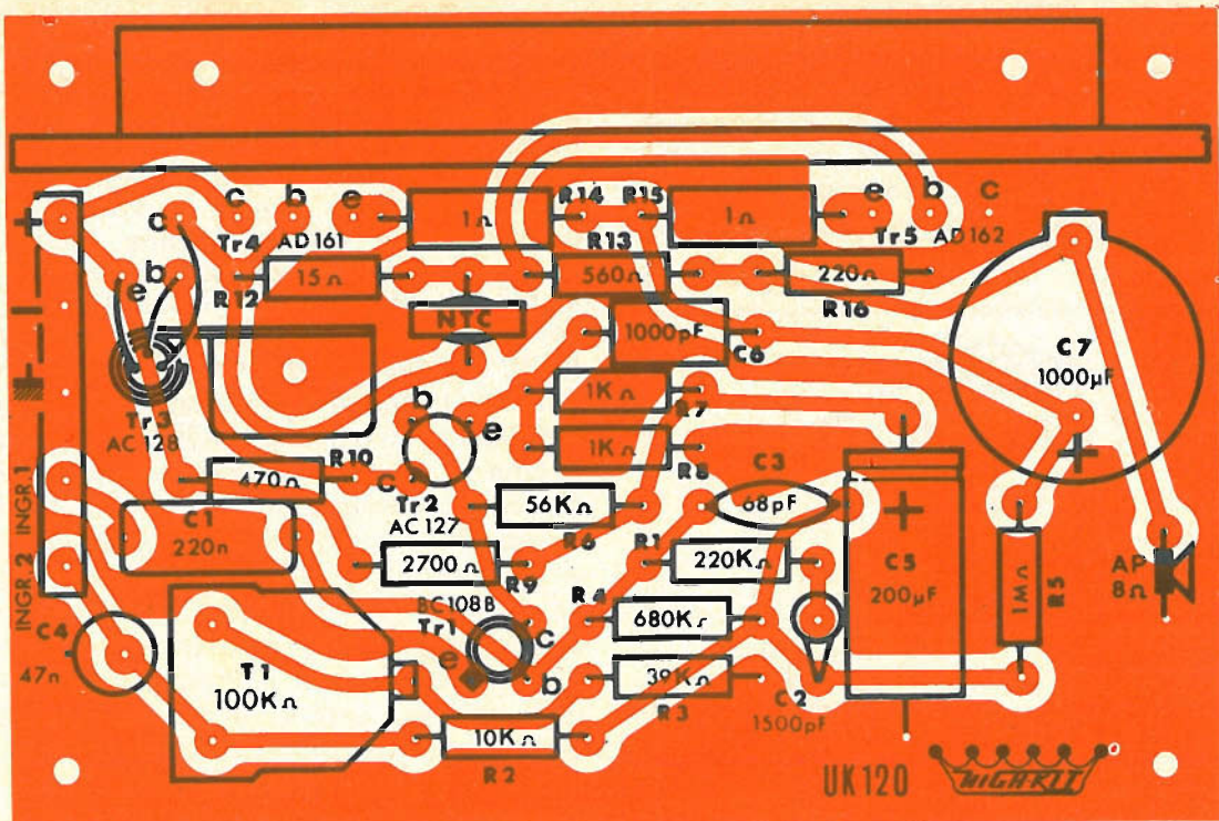
Fig. 2 - Vista serigrafica della basetta a circuito stampato.
