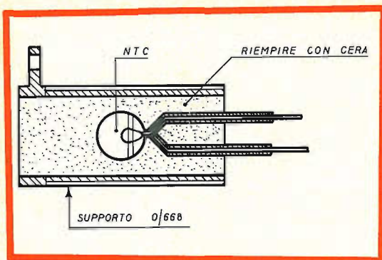
Fig 3 - L'elemento NTC inserito nel suo supporto
