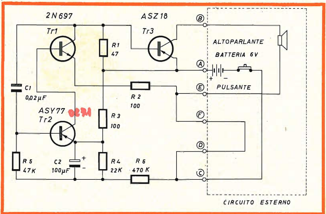
Fig. 1 - Schema di principio del circuito elettrico.
