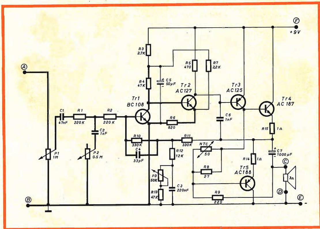
Fig. 1 - Schema elettrico dell'apparecchio.
