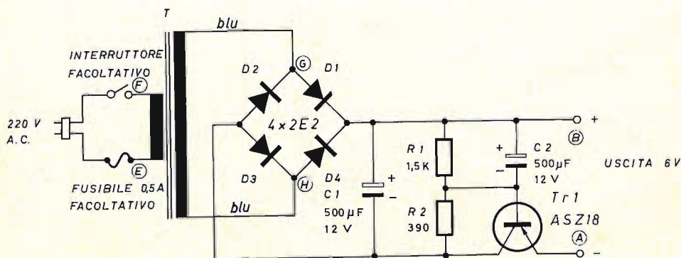
Fig. 1 - Schema di principio del circuito elettrico.
